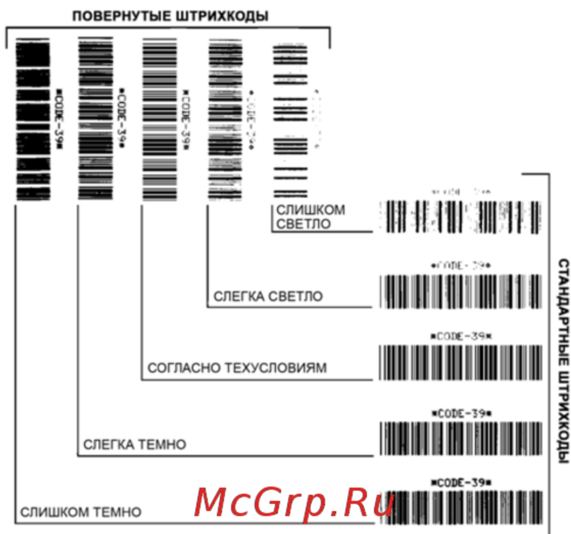
Рис. 3 • Сравнение темности штрихкодов
