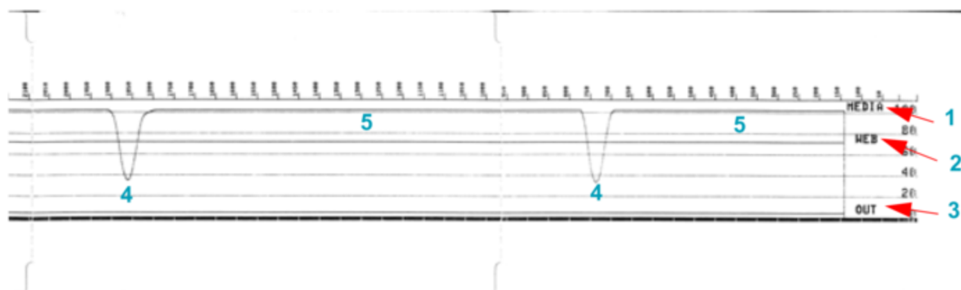
Рис. 6 • Профиль датчика (носитель с черными метками)
